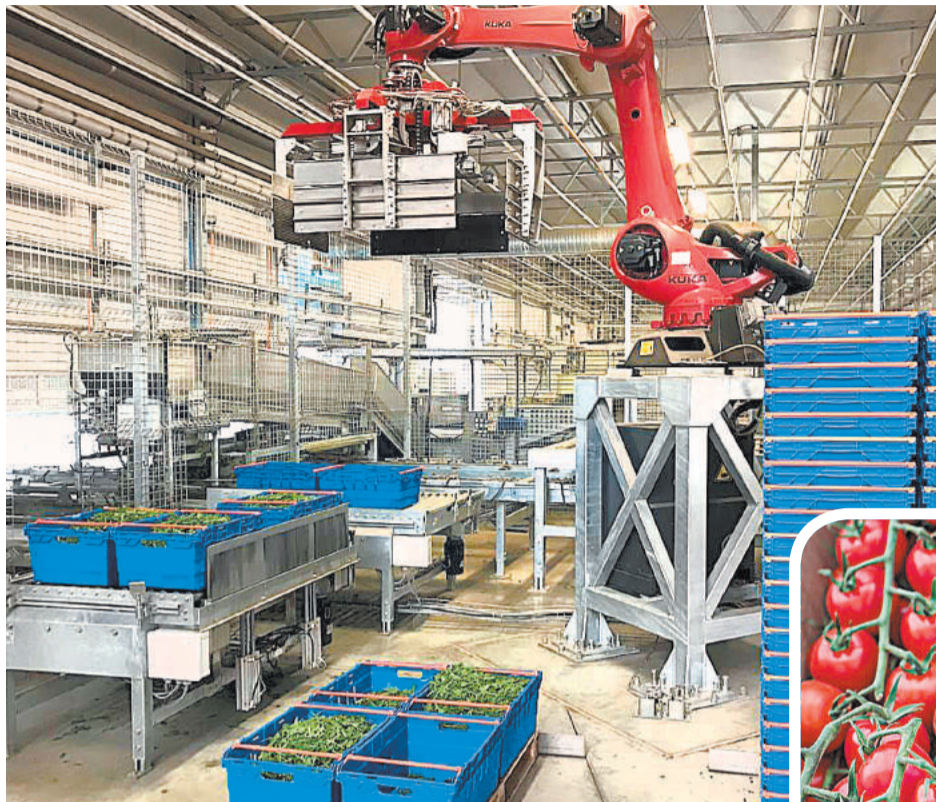
Робот составляет коробки с зеленью на тележки, а те сами отвозят их на упаковочную линию.
